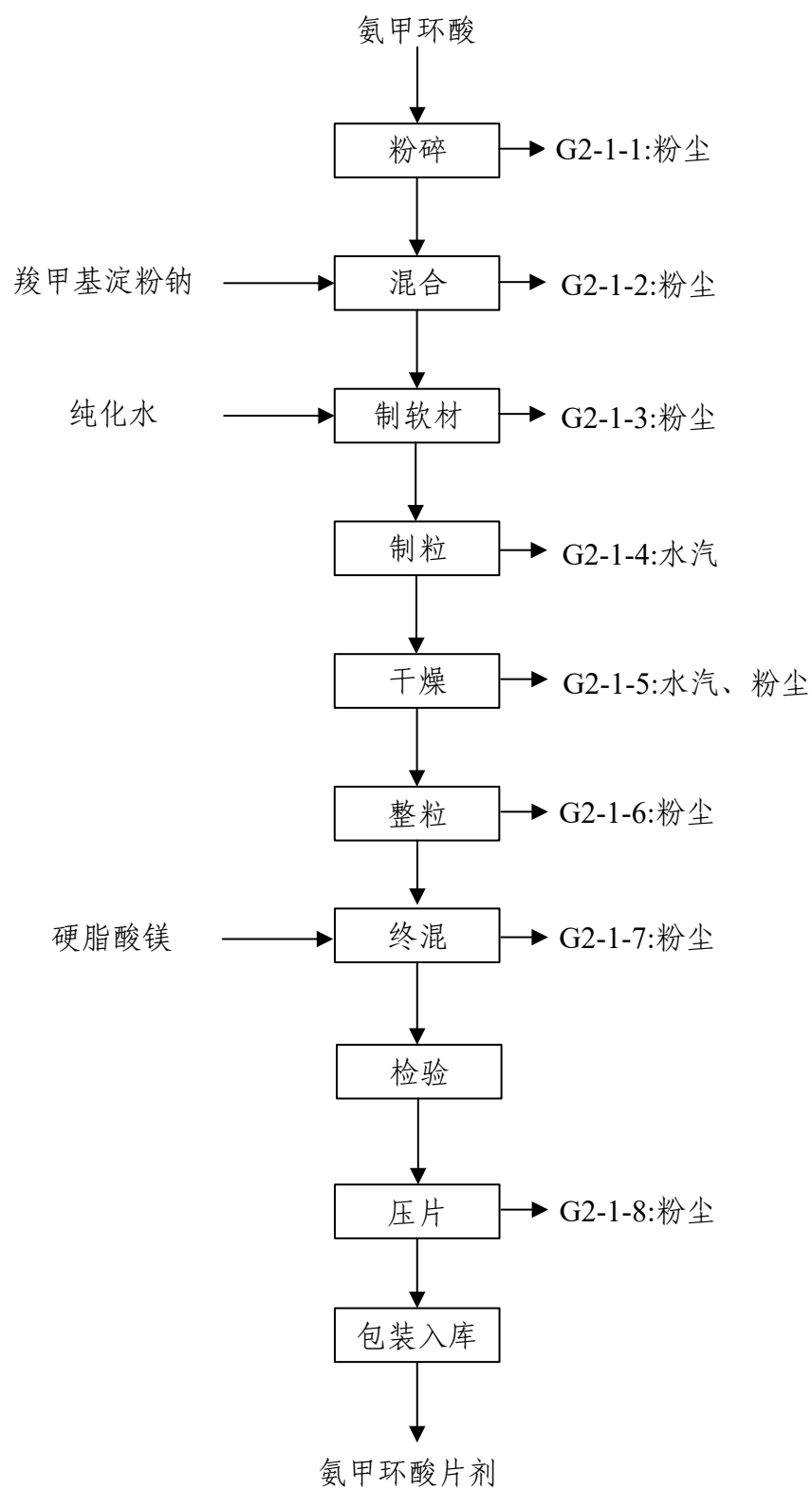
图 2.1-1 氨甲环酸片剂生产工艺流程图
